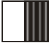
2 Door Robe 150cm(W) x 67cm(D) x 217cm (H)
