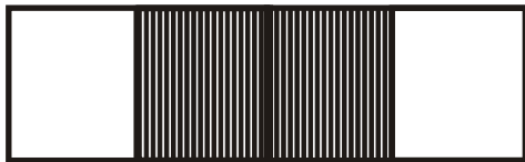
4 Door Robe - Synchronous Opening 400cm(W) x 67cm(D) x 217cm (H)
